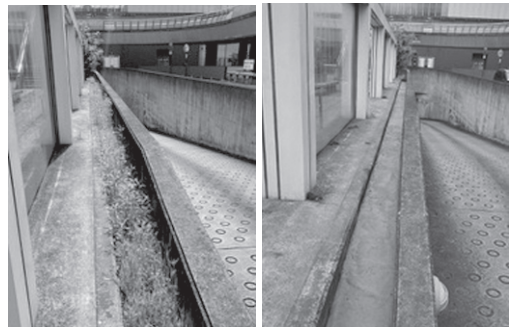
JR奈良駅構内の側溝に生えた雑草(左)の根と土を固め、青く着色した「塗るNAOS(ナオス)」で仕上げ(右)
